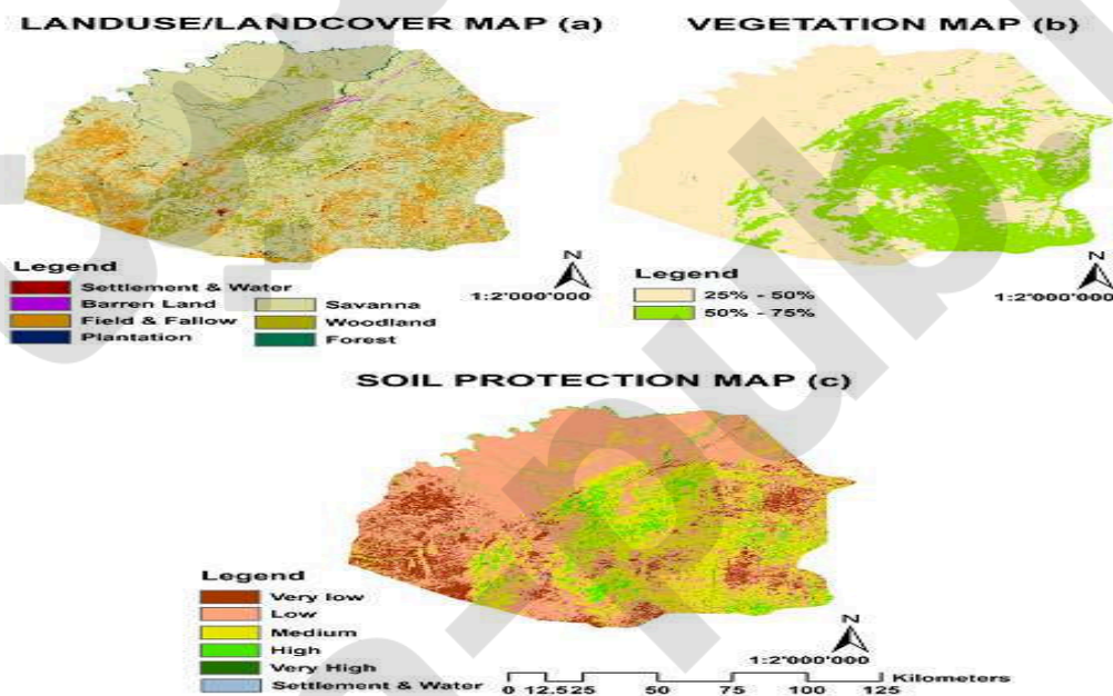
شکل 4. نقشه پوشش استفاده از زمین (A)، پوشش گیاهی (ب) (پوشش گیاهی مخفف کسری از زمین تحت پوشش گیاهی سبز)، حفاظت از خاک (ج).
