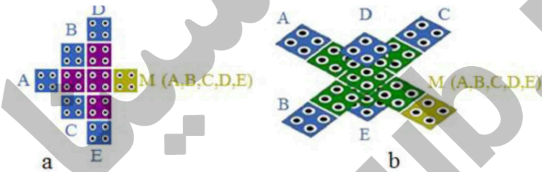
شکل 6: مناطق زمان سنج در فناوری QCA {18}
