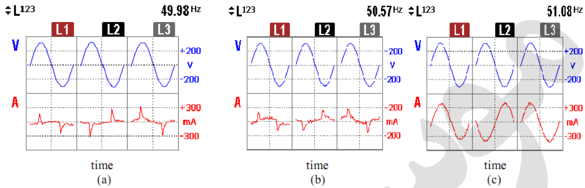
شکل 2- ویژگی های جریان و ولتاژ به دست آمده در طی ساختار آزمایشی با استفاده از الف- فناوری ال ایی دی ب- فناوری سی اف ال و ج- فناوری رشته ای
